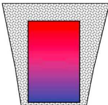
Figura 6.27 – Distribuția optimă neomogenă a izolației (conf. cu Dahash et al)
