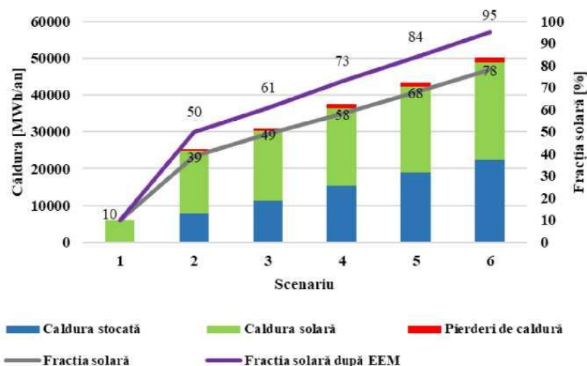
Figura 6.28 – Căldura din rețeaua de încălzire centralizată cu energie solară și fracția solară pentru scenariile analizate (cf. cu Soloha et al., 2017)
