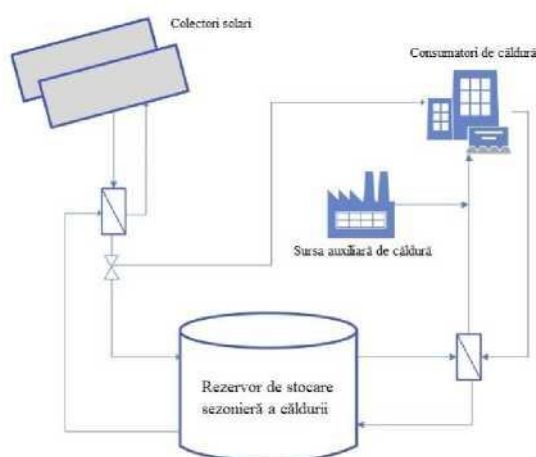
Figura 6.20 - Configurația sistemului centralizat de încălzire solară cu stocare sezonieră de căldură (conf. cu Soloha et al., 2017)
